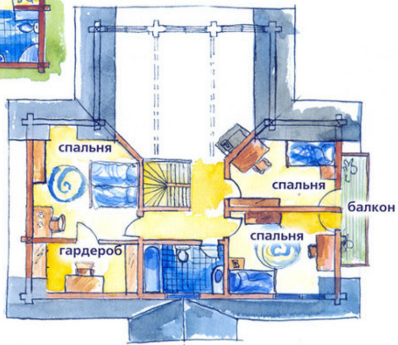
план 2 этажа
