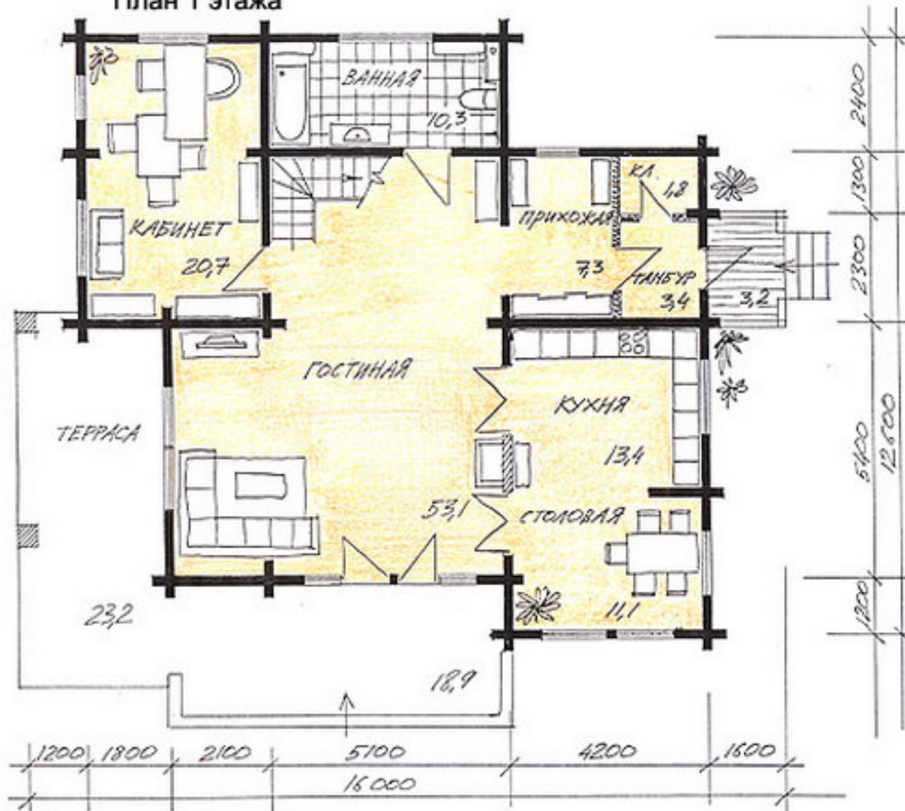
План 1 этажа
