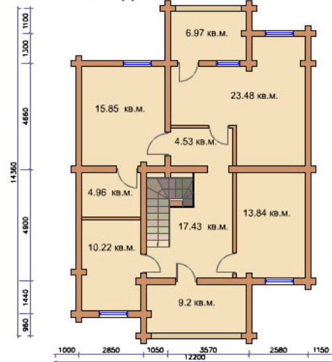
ПЛАН МАНСАРДЫ
