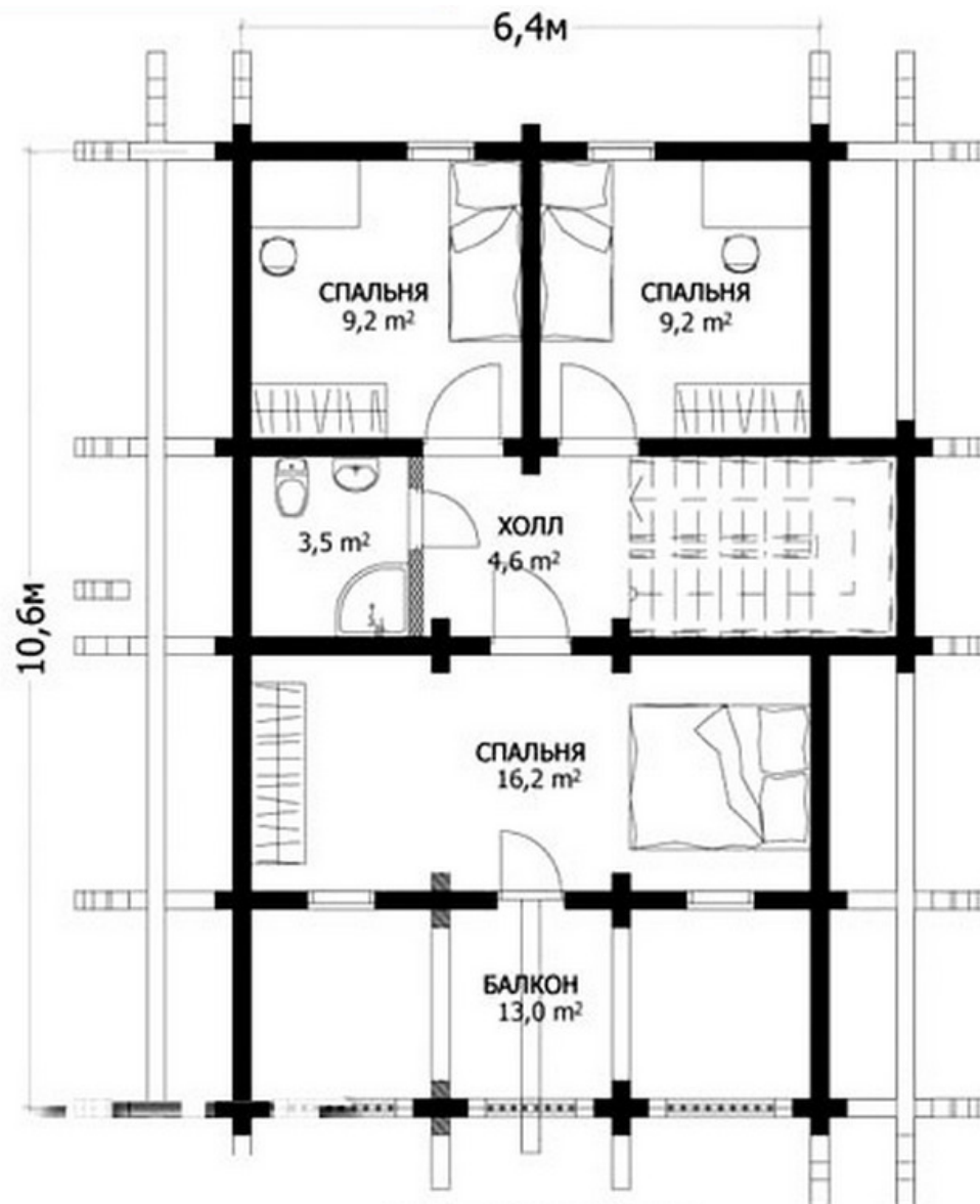
ПЛАН МАНСАРДЫ
