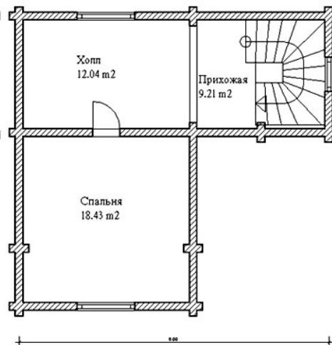
ПЛАН МАНСАРДЫ
